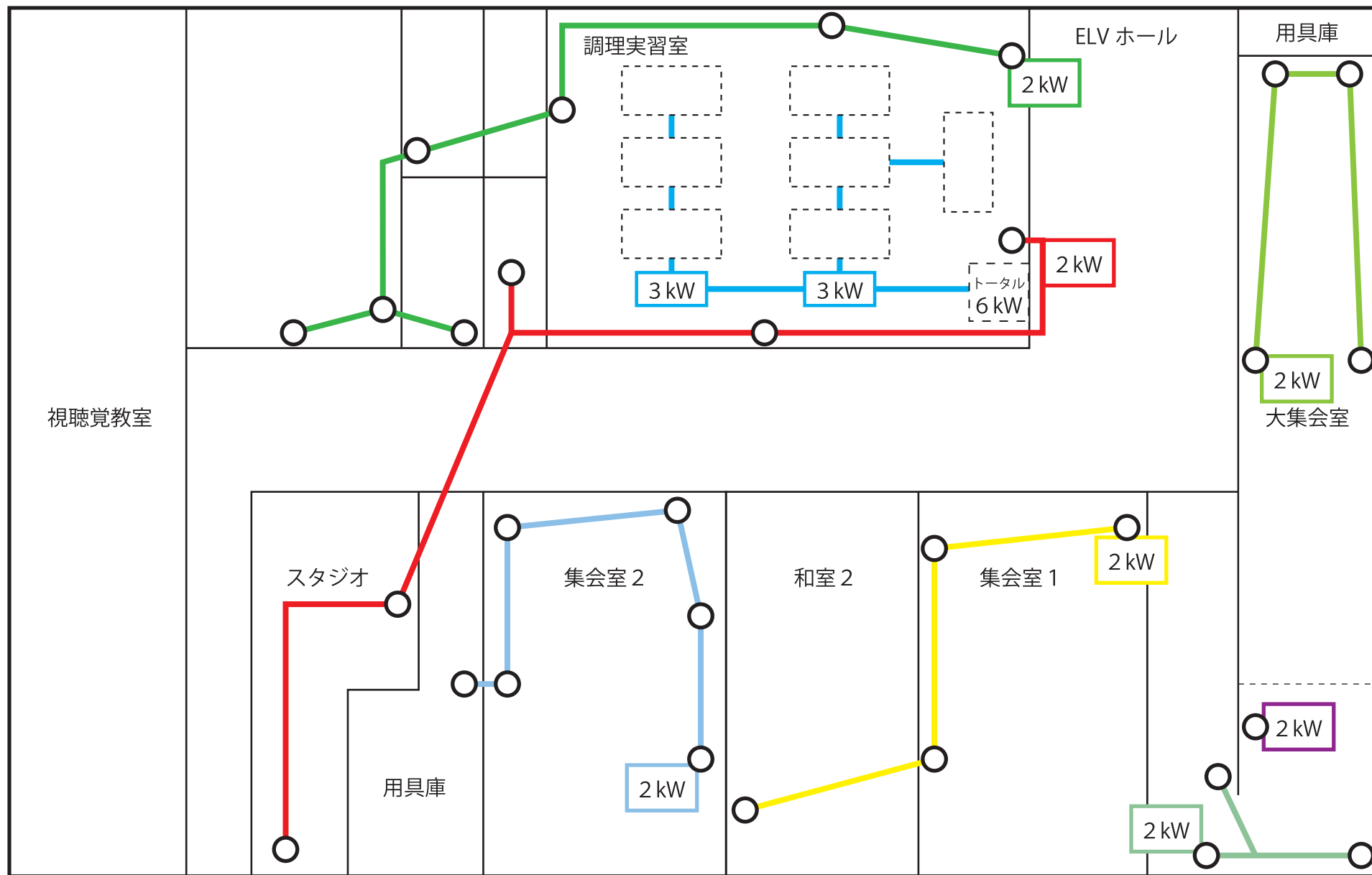
館内コンセント容量及び系統図 2F
